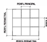
MÓDULO ESTÁNDAR GRILLA 1000 x 1000 mm. A EJE
