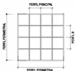
MÓDULO ESTÁNDAR GRILLA PARA CIELO CELL 671 x 671 mm. A EJE
