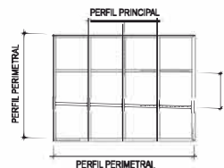
MÓDULO ESTÁNDAR GRILLA PARA CIELO CELL 671 x 671 mm. A EJE
