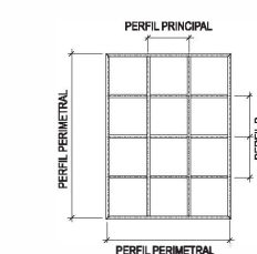
MÓDULO ESTÁNDAR GRILLA PARA CIELO TILE LAY-IN 645 x 645 mm. A EJE
